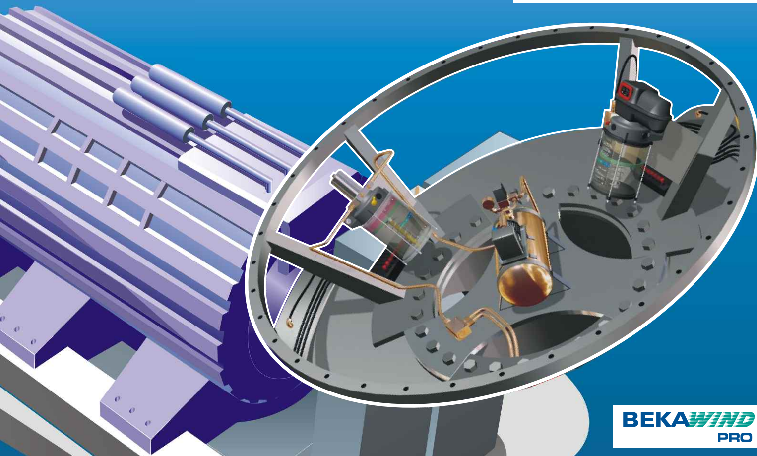
Blattlager mit Progressivverteiler und Entsorgungsbehälter
